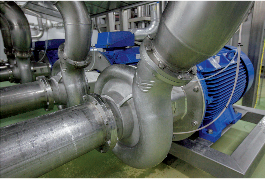
Die Strömungsoptimierung und die daraus resultierende Energieeinsparung werden im Wesentlichen durch ein gegossenes Spiralgehäuse erreicht
